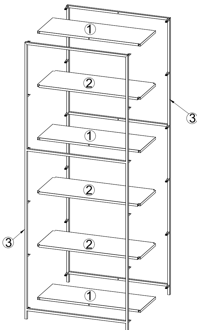
Teileliste
